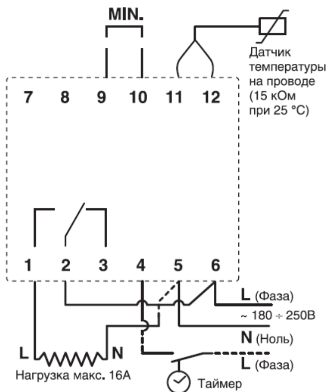
Рис.2. Схема подключения Devireg ™ 316.
